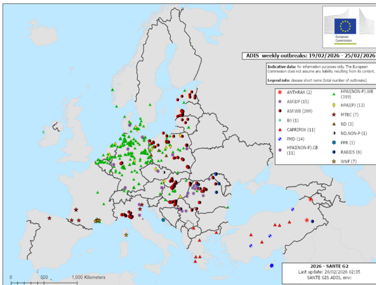
Карта1: Обявените заболявания за периода 19.02. - 25.02.2026 г. по данни на ADIS в ЕС.
