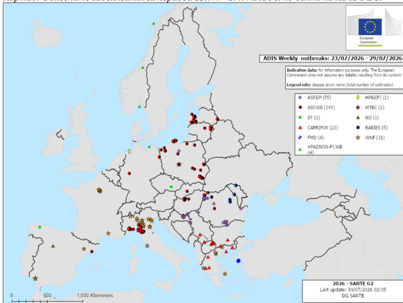
Карта1: Обявените заболявания за периода 23.07. – 29.07.2026 г. по данни на ADIS в ЕС.
